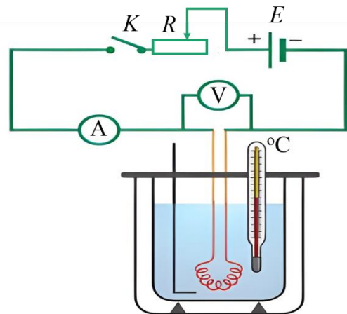
Hình 7. Sơ đồ thí nghiệm đo nhiệt dung
