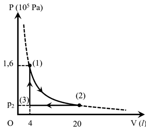
Hình II.1. Đồ thị quá trình biến đổi trạng thái (1) → (2) → (3)
