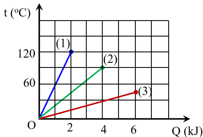
Hình I.3. Đồ thị độ biến thiên nhiệt độ theo nhiệt lượng cung cấp
