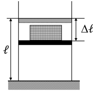
Hình II.2. Xi lanh chứa khí
