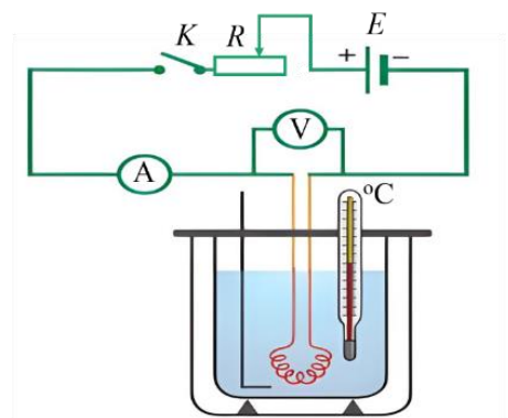
Hình 7. Sơ đồ thí nghiệm đo nhiệt dung
